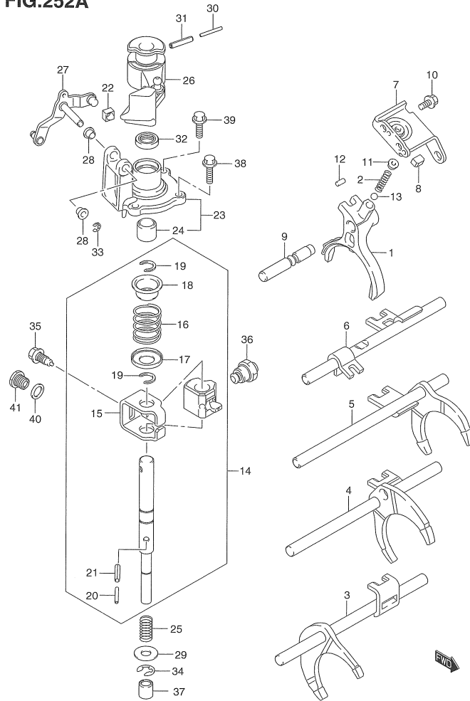
ZC33S 252A MT GEAR SHIFT FORK
